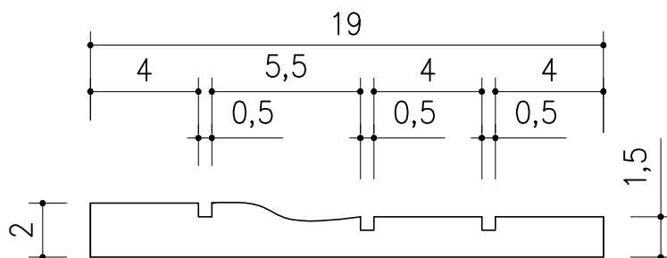
RAMKA OKIENNA – PRZEKRÓJ
