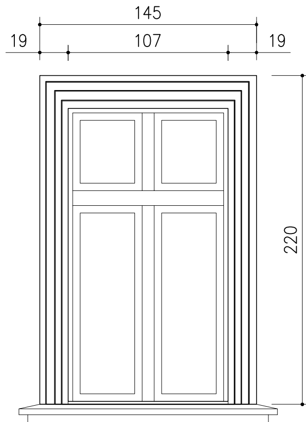
WIDOK OBRAMOWANIA OKNA
