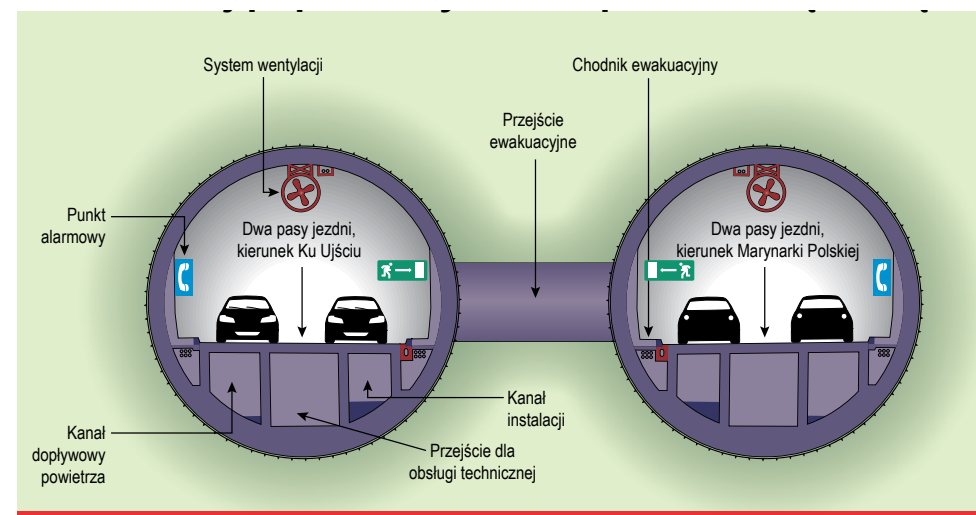
Przekrój poprzeczny tunelu pod Martwą Wisłą
