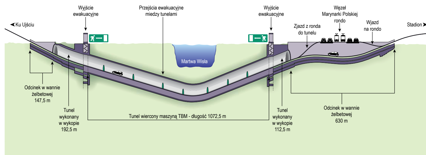
Przekrój podłużny tunelu pod Martwą Wisłą
