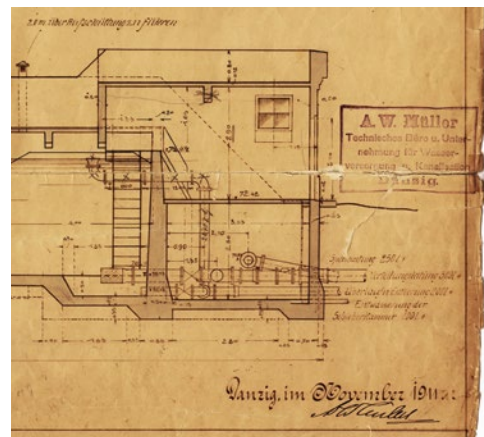
Fragment oryginalnej dokumentacji zbiornika Stara Dolina (1911 r.).
