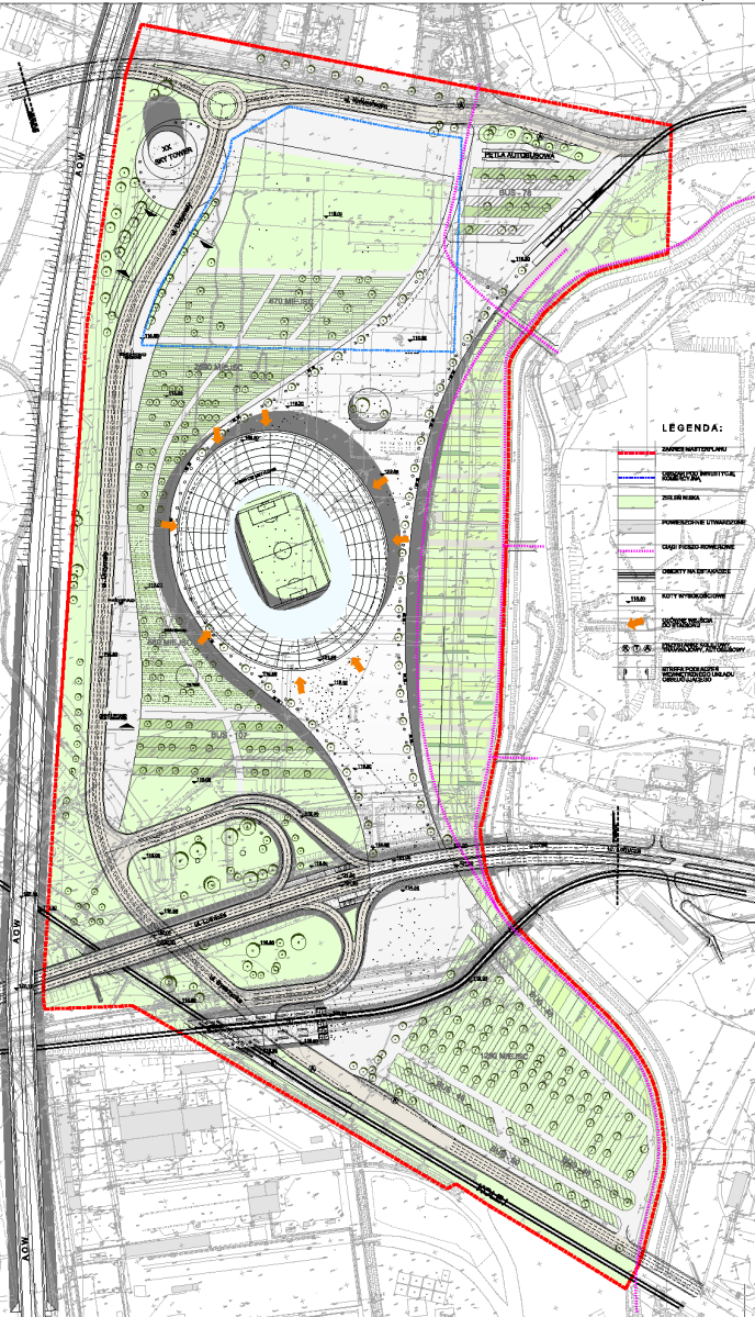
masterplan wersja A bez uwzględnienia centrum komercyjnego, widok z góry
