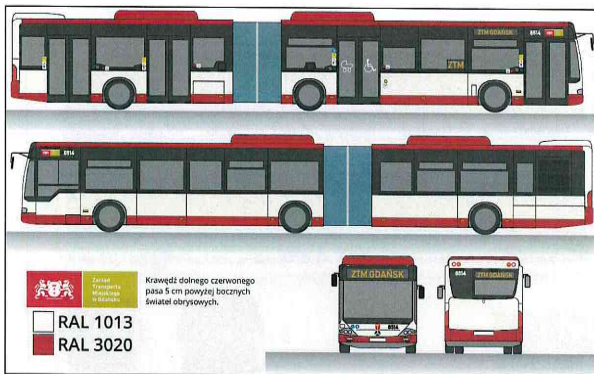
Rys. 12.7.3. Mercedes Conecto G Euro 6
