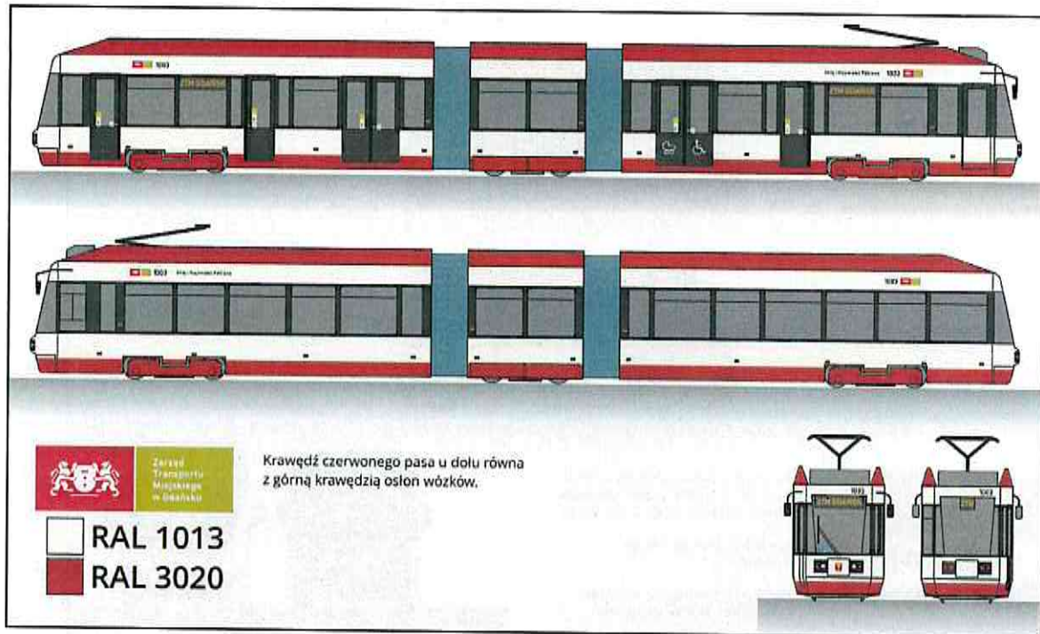
Rys. 12.3.4. Alstom NGd99
