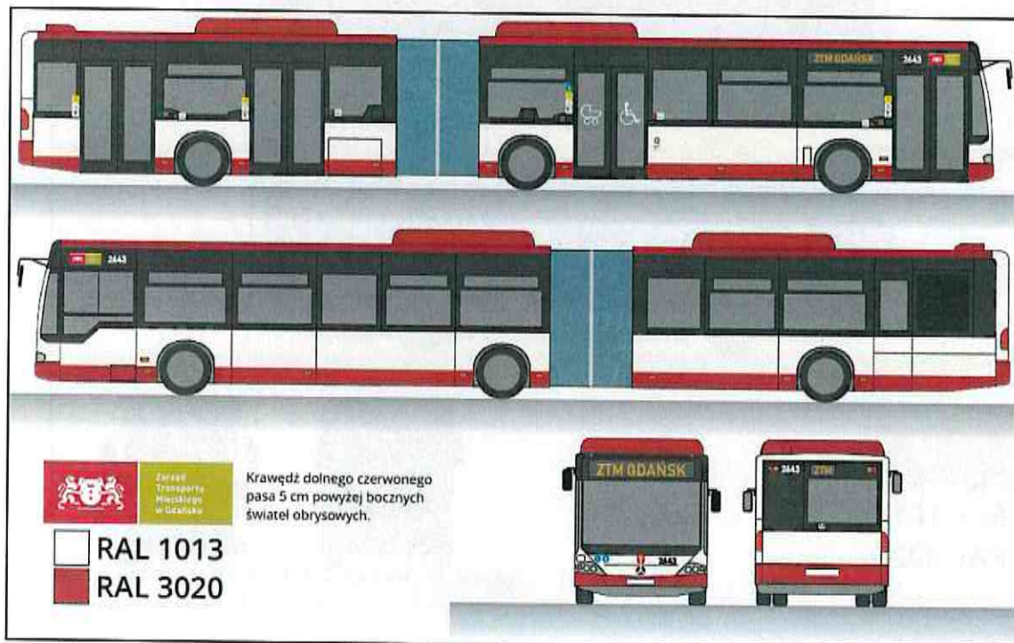
Rys. 12.7.2. Mercedes Conecto G EEV
