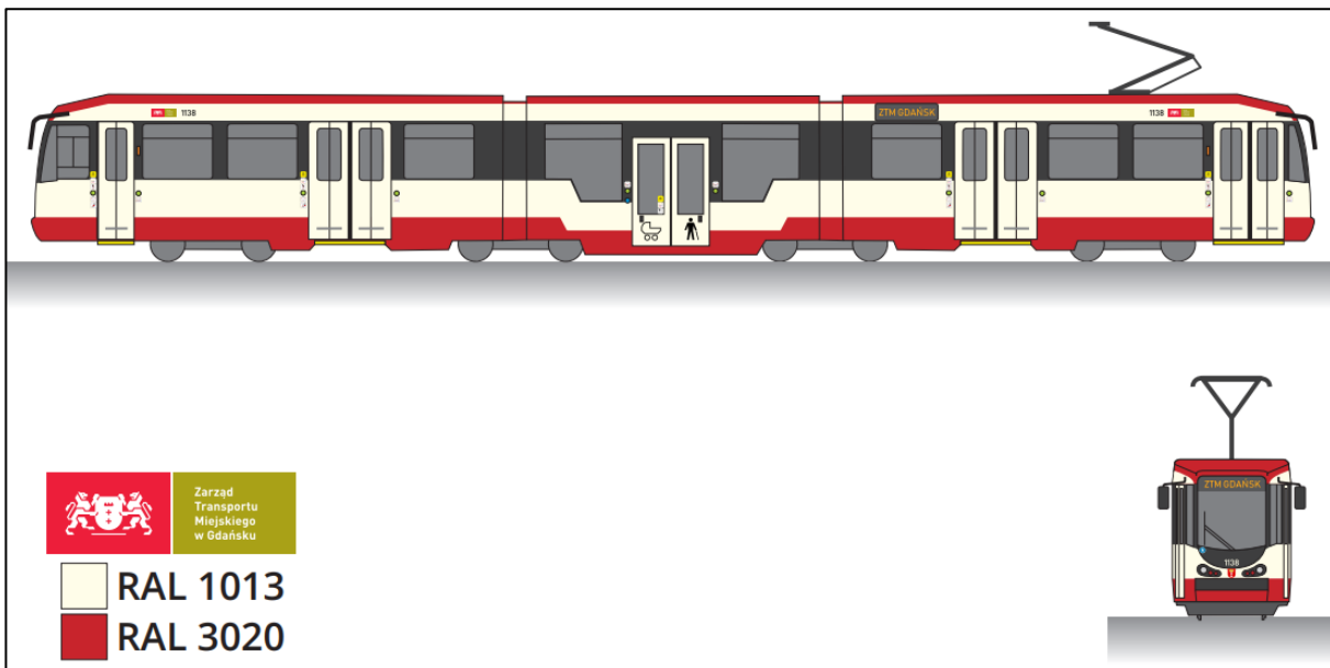
Rys. 12.2.1. Düwag N8C
