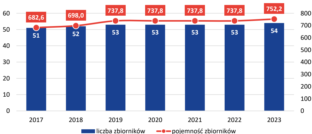
Liczba i pojemność zbiorników przeciwpowodziowych i retencyjnych w Gdańsku w latach 2017–2023 - dane w szt. i tys. m 3 -
