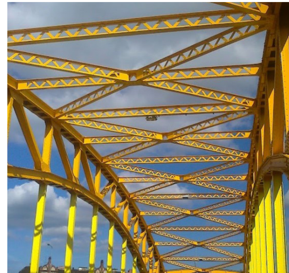
istniejący w sąsiedztwie "Żółty Wiadukt" z widocznymi stężeniami kratowymi
