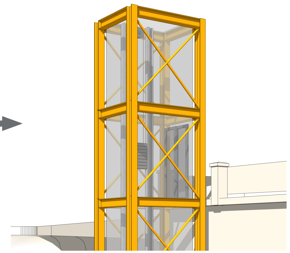
wykorzystanie motywu stężeń w projektowanej konstrukcji szybu windowego
