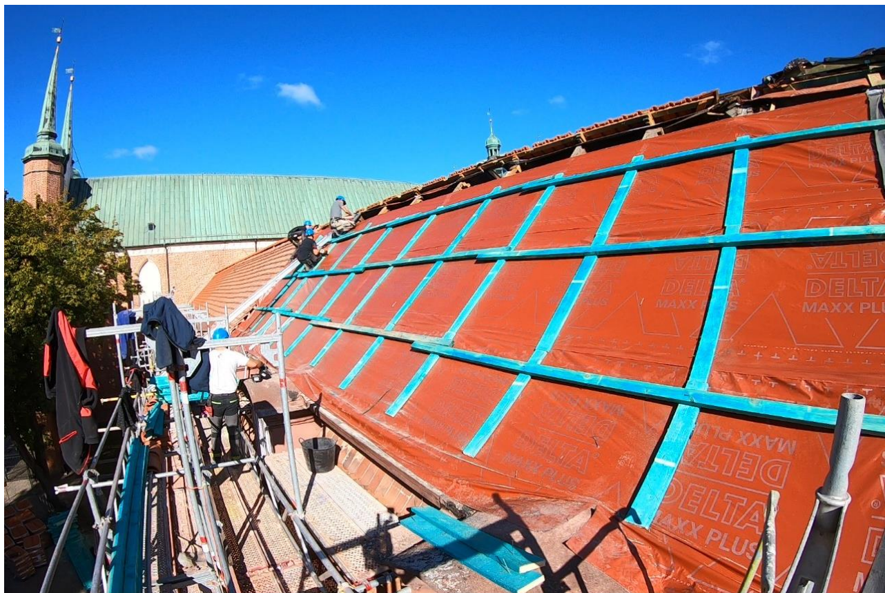
Ilustracja 34. Montaż membrany paroprzepuszczalnej i łączenia
