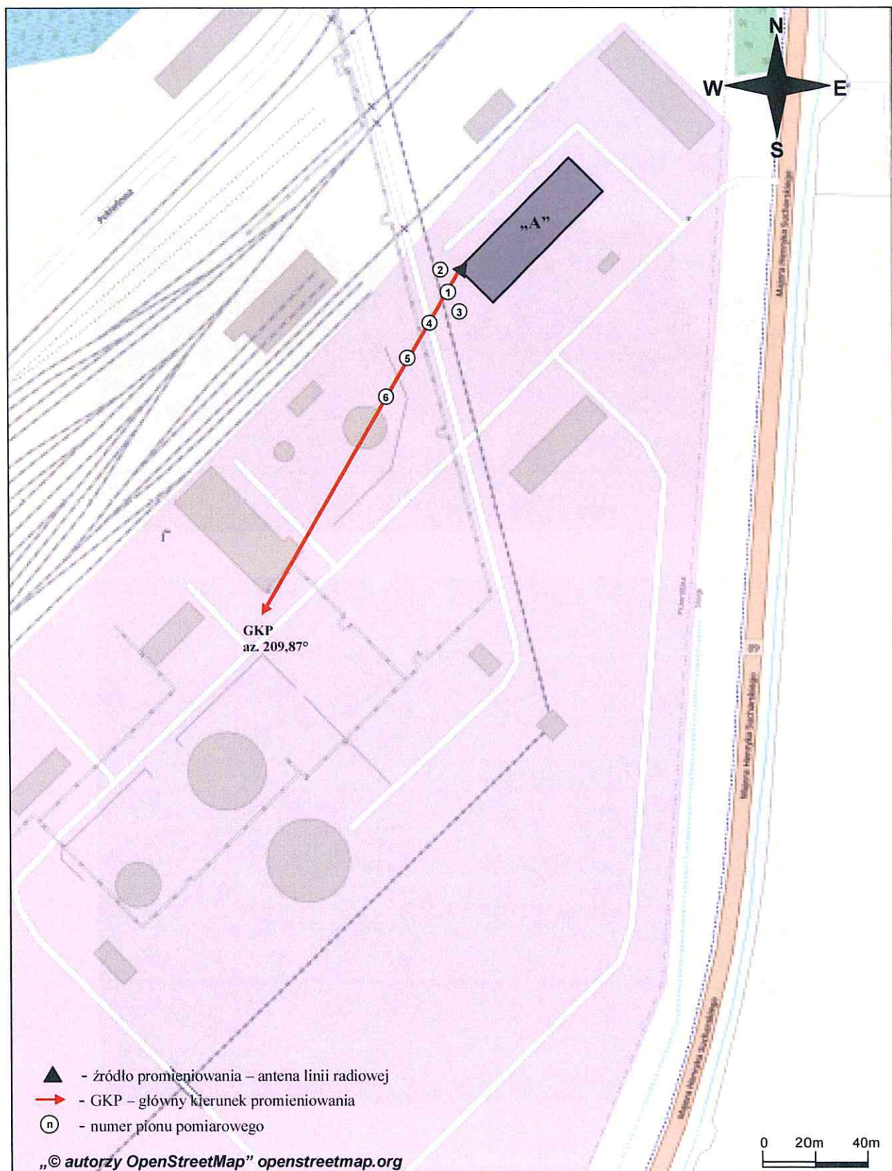
Rys. 1. Usytuowanie punktów i pionów pomiarowych w otoczeniu instalacji radiokomunikacyjnej Stacja Netia GDANB167-GDANM00386 Gdańsk, ul. mjr. Henryka Sucharskiego 12
