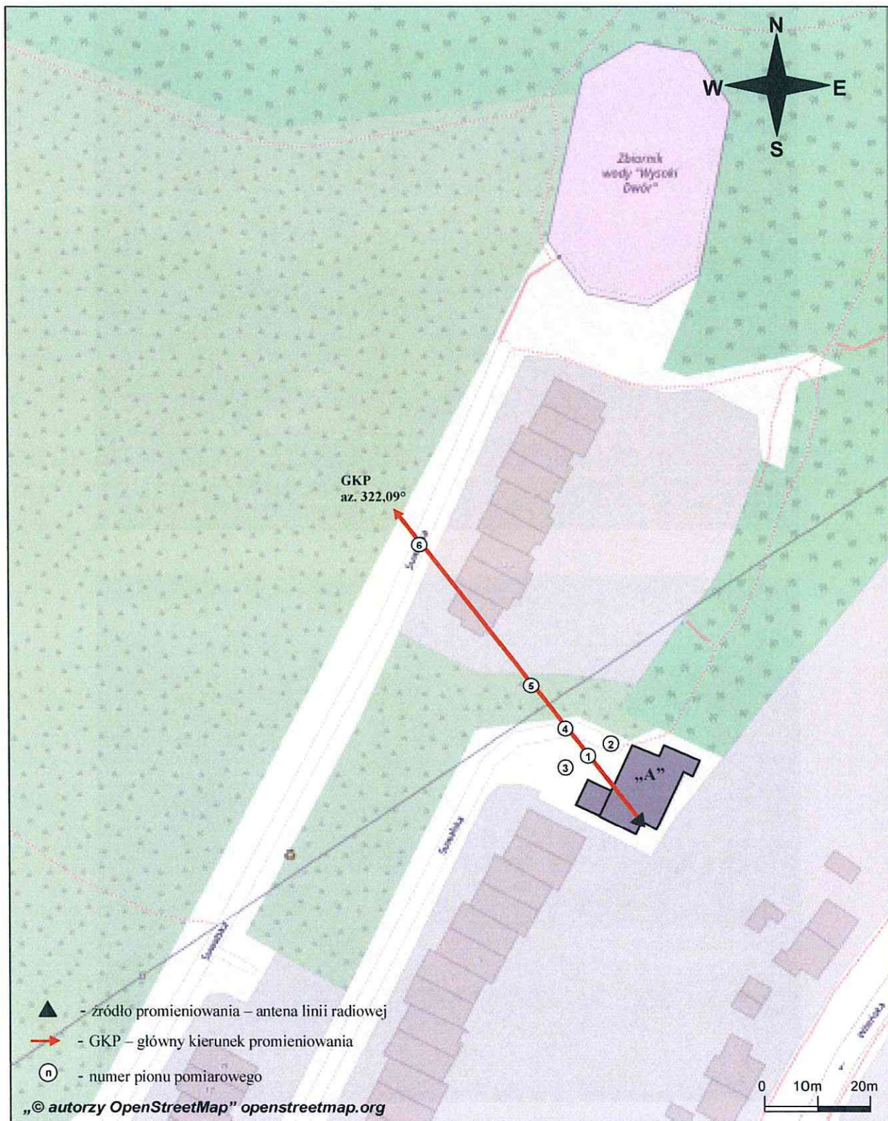
Rys. 1. Usytuowanie punktów i pionów pomiarowych w otoczeniu instalacji radiokomunikacyjnej Stacja Netia GDAND503-GDANM00425 Gdańsk, ul. Suwalska 46
