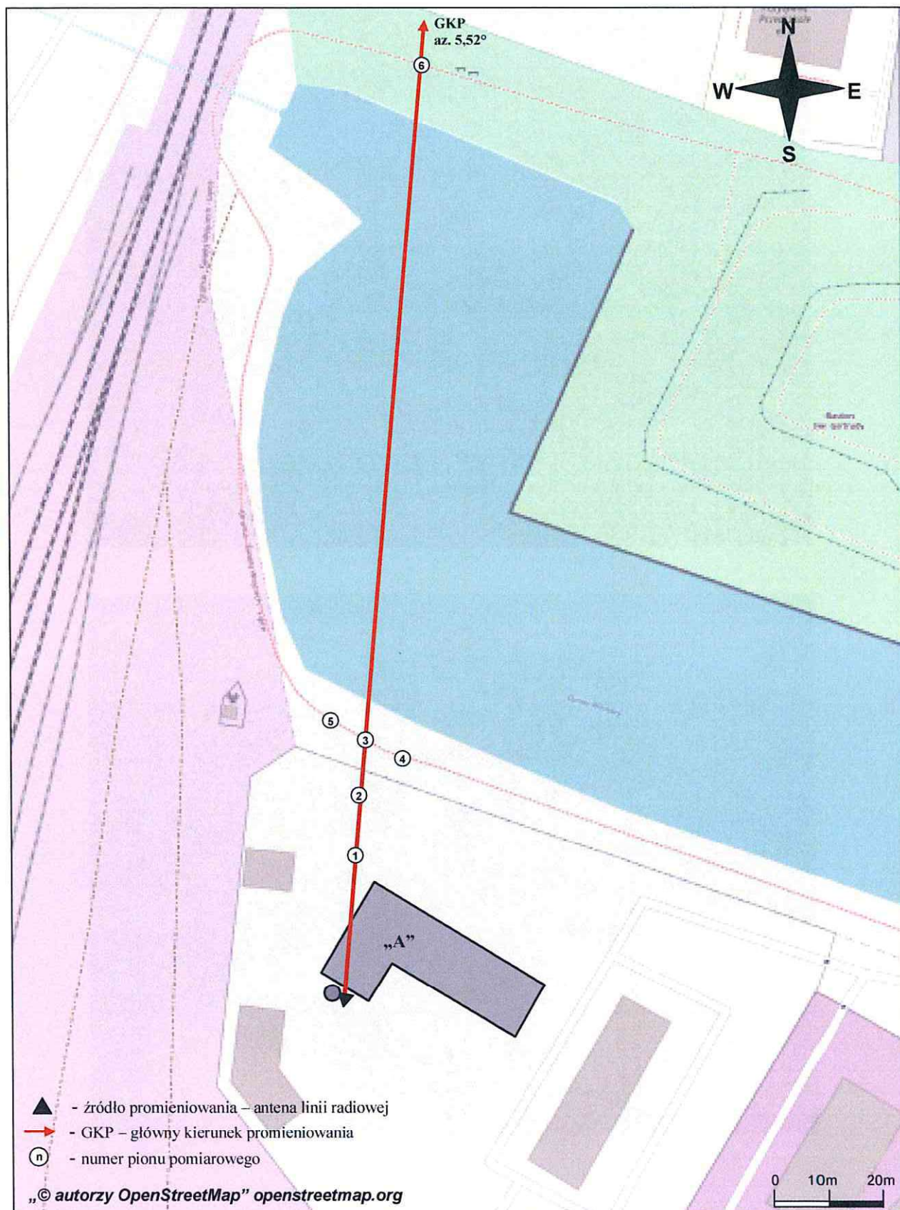
Rys. 1. Usytuowanie punktów i pionów pomiarowych w otoczeniu instalacji radiokomunikacyjnej Stacja Netia GDAFB067-GDANM00440 Gdańsk, ul. Mostowa 1
