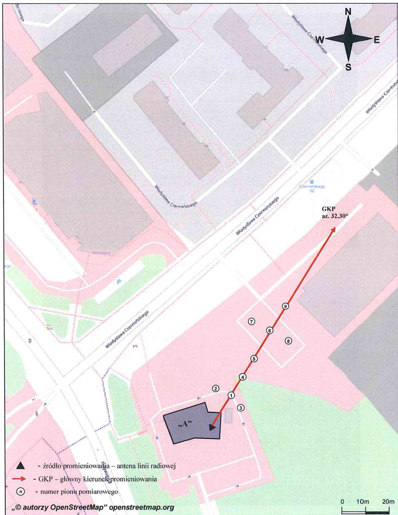
Rys. 1. Usytuowanie punktów i pionów pomiarowych w otoczeniu instalacji radiokomunikacyjnej Stacja Netia GDAND364-GDANM00409 Gdańsk, ul. Przywudzka 11
