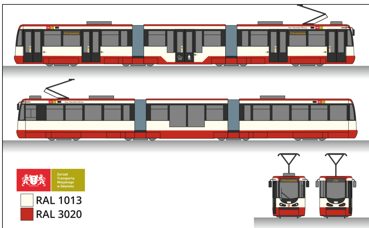
Rys. 12.2.2. Konstal typ 114Na (1501)
