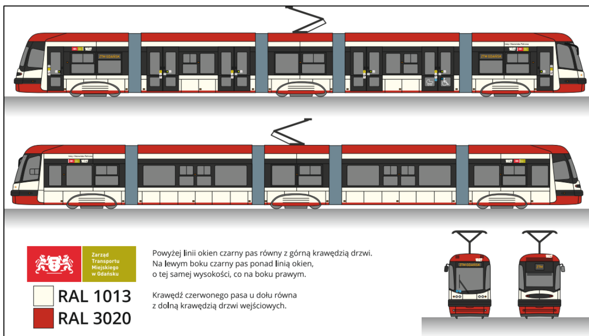
Rys. 12.3.2. Pesa Swing
