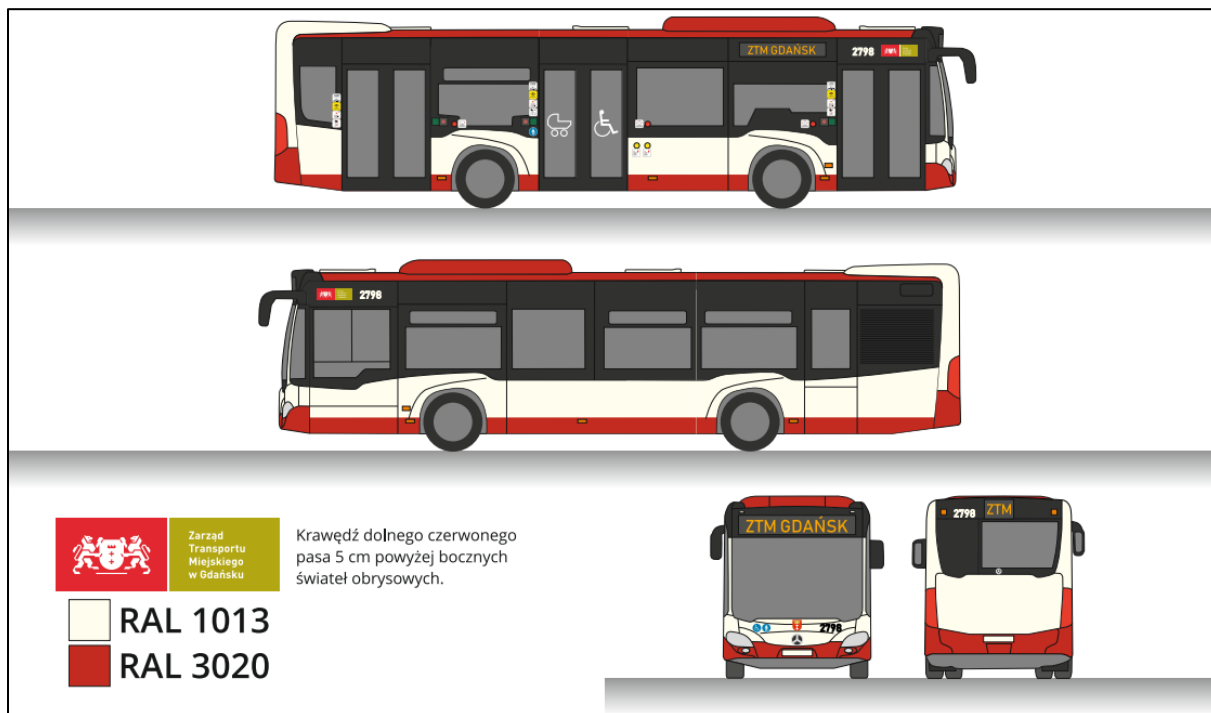
Rys. 12.5.1. Mercedes Citaro K C2
