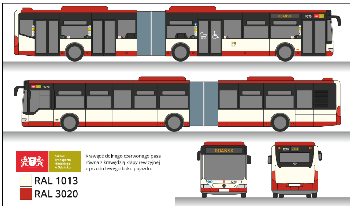
Rys. 12.7.4. Mercedes Citaro G II (Lift)
