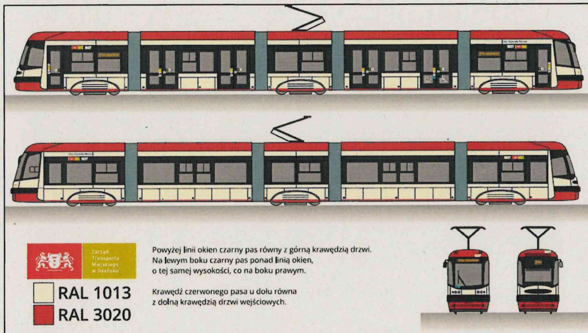
Rys. 12.3.2. Pesa Swing
