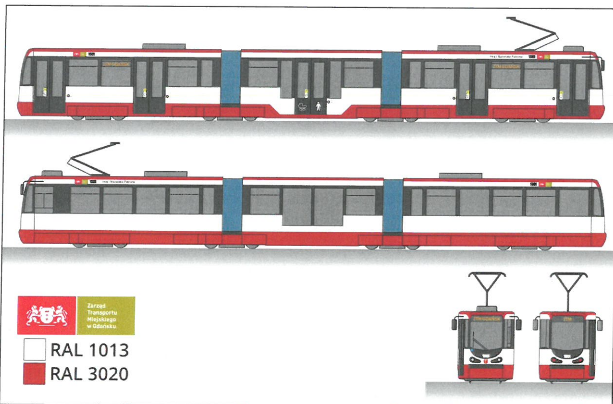
Rys. 12.2.2. Konstal typ 114Na (1501)
