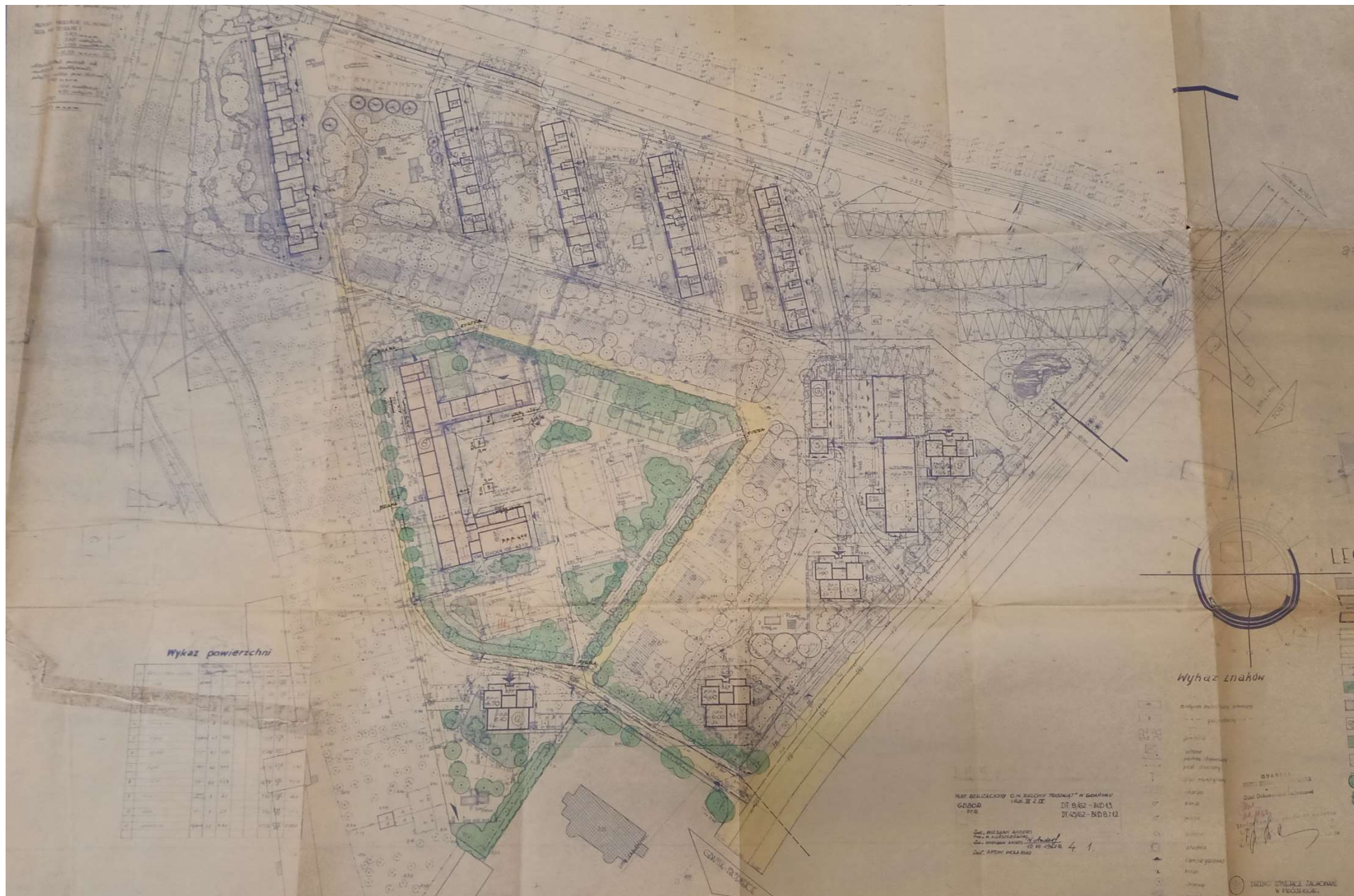
15) Fragment „Planu realizacyjnego – Osiedle mieszkaniowe Zielony Trójkąt” (1962 r.) opracowanego przez architektów W.Andersa i H.Kleszczewskiego. Widoczne skupienie projektowanej zabudowy na północnym i wschodnim obrzeżu zespołu oraz planowane pozostawienie dużej części oryginalnej zabudowy wraz z charakterystycznym trójkątnym układem wewnętrznego kwartału. (źródło: zbiory Archiwum Wydziału Architektury Urzędu Miejskiego w Gdańsku)
