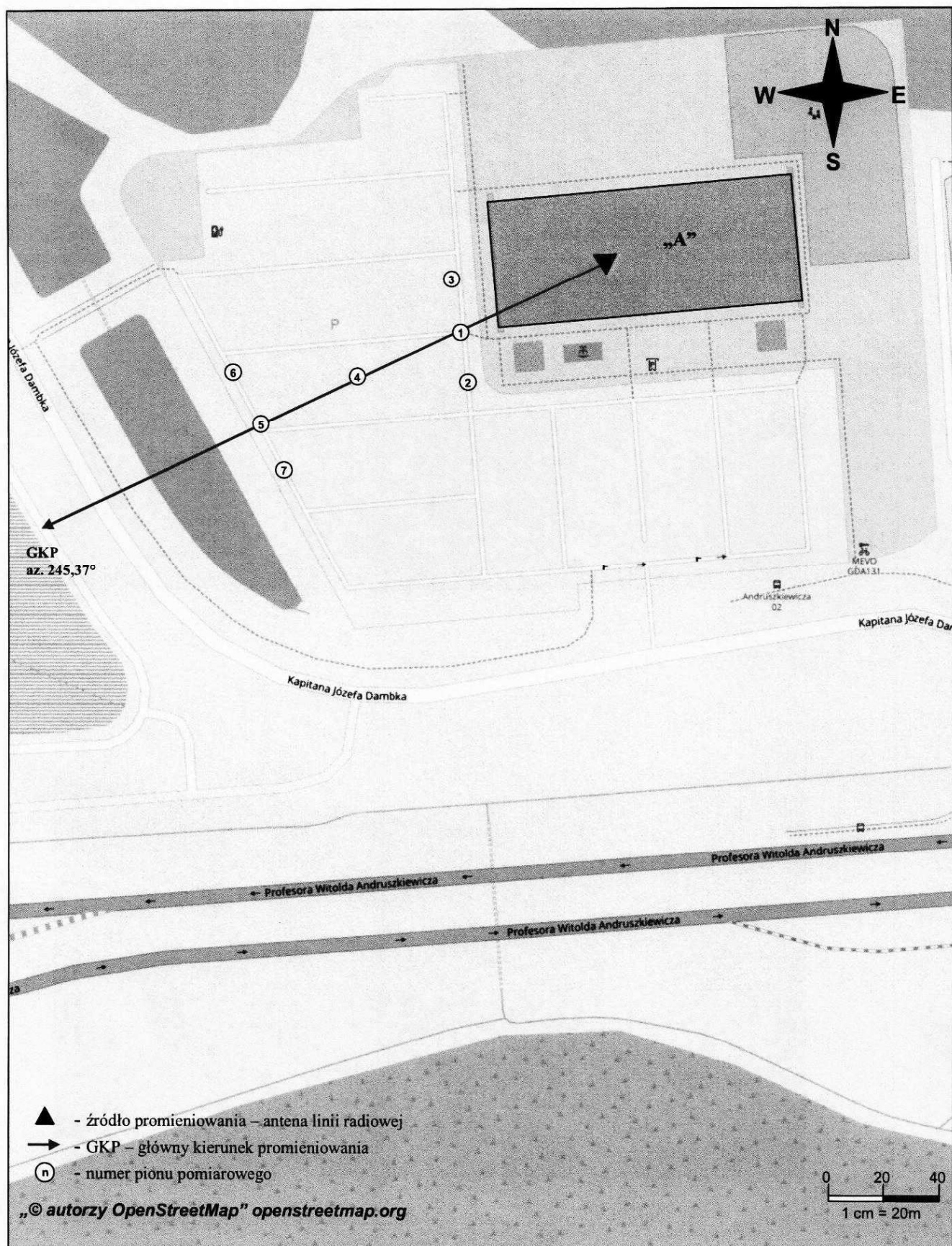
Rys. 1. Usytuowanie punktów i pionów pomiarowych w otoczeniu instalacji radiokomunikacyjnej Stacja Netia GDANB941-GDANM00376 Gdańsk, ul. prof. Witolda Andruszkiewicza 5
