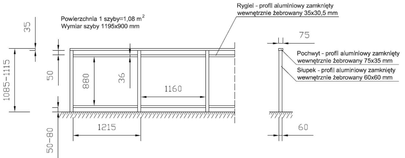
Rys. 11 Wygradzenie typu RS
