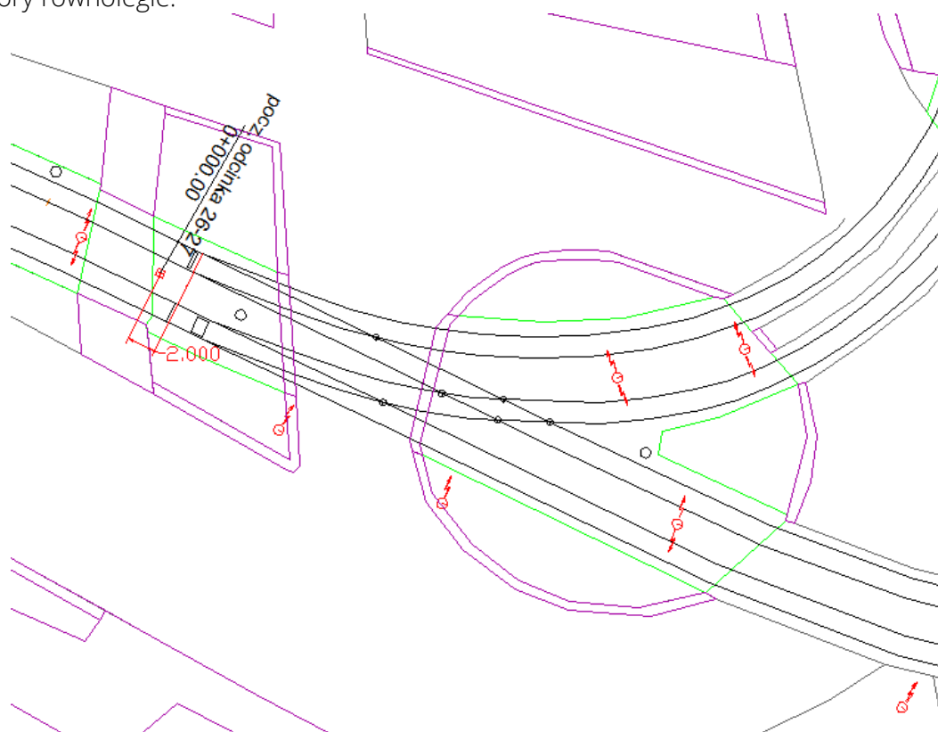
Rys. 1 Punkt umowny początku i końca odcinka międzywęzłowego
