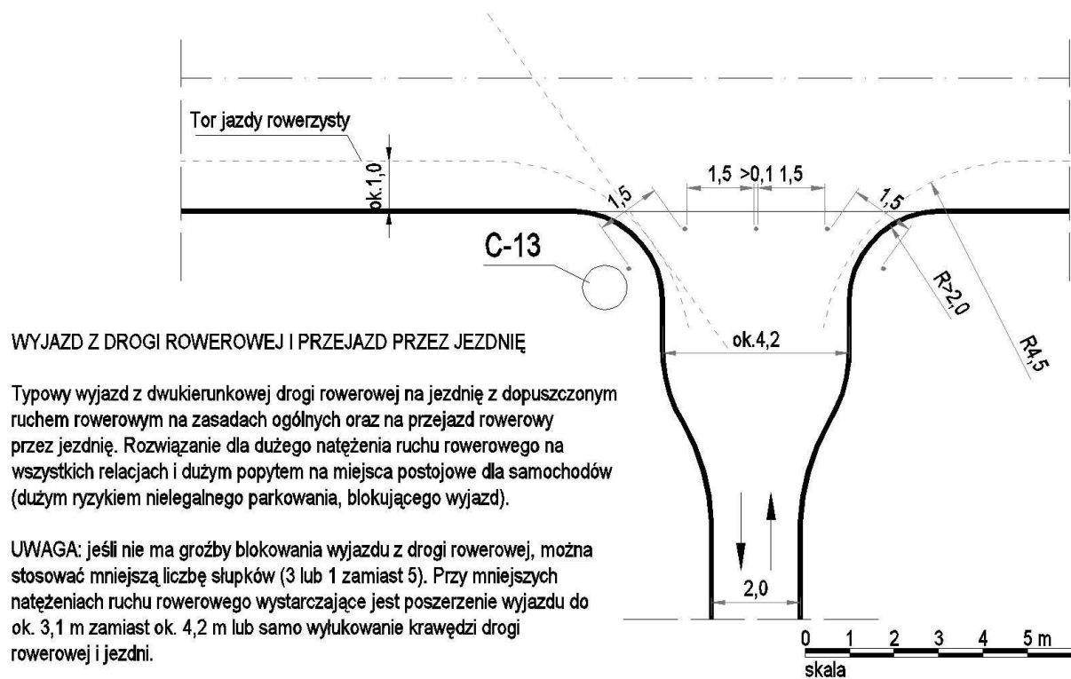
Rysunek 13 Wyjazd z drogi rowerowej - przypadek 2
