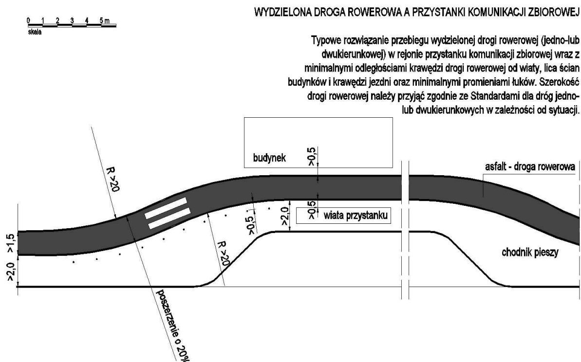
Rysunek 23 Optymalna lokalizacja drogi rowerowej w rejonie przystanku autobusowego
